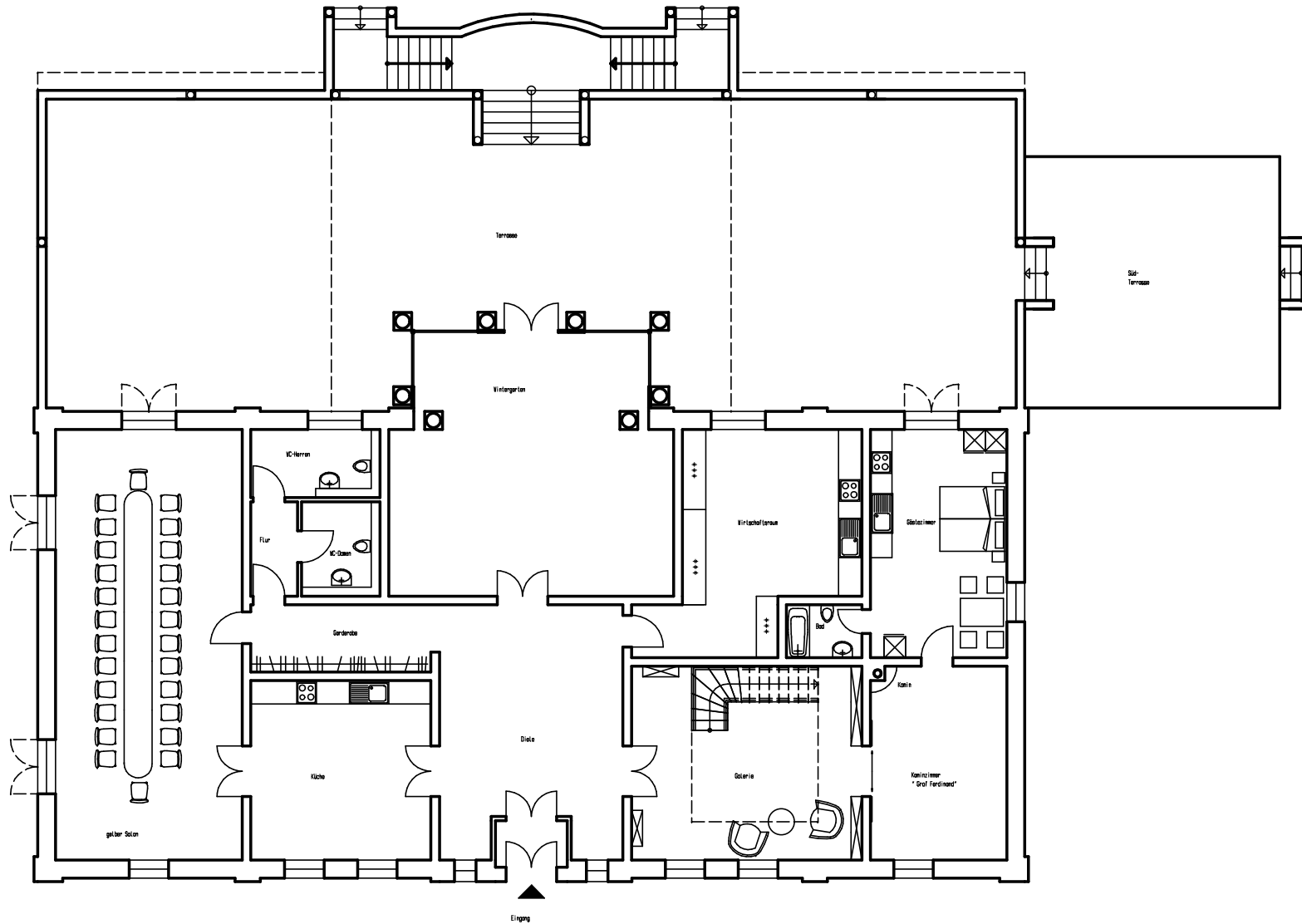
Erdgeschoss M 1:175
